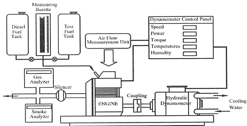
รูปที่ 1 ชุดอุปกรณ์การทดสอบและการติดตั้งเครื่องมือวัด
