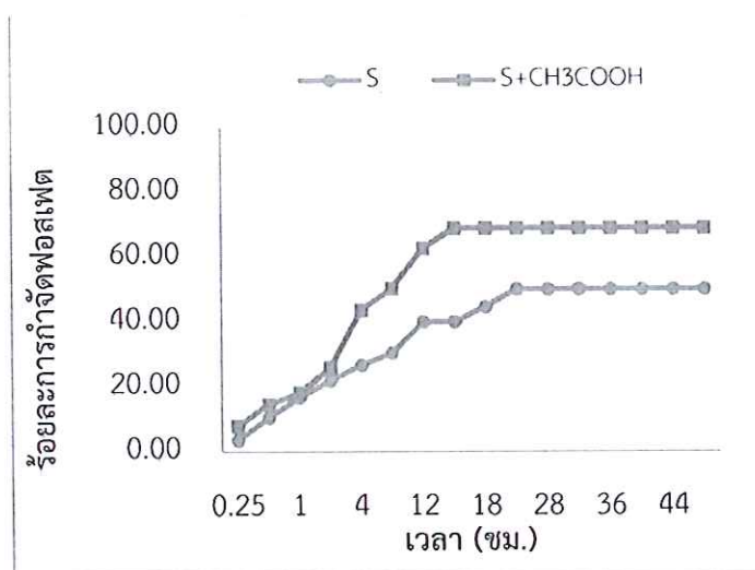
รูปที่ 4 ระยะเวลาสมดุลของการดูดซับฟอสเฟตของตัวดูดซับที่ไม่ได้กระตุ้น (S) และกระตุ้นด้วยกรดอะซิติก ( S+CH_3COOH )
