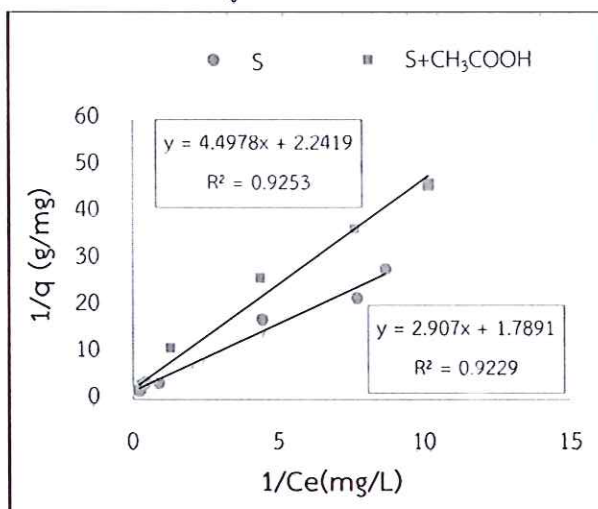
รูปที่ 5 Langmuir Adsorption Isotherm ของตัวดูดซับที่กระตุ้นและไม่กระตุ้นกรดอะซิติก
