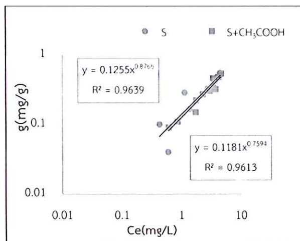
รูปที่ 6 Freundlich Adsorption Isotherm ของตัวดูดซับที่กระตุ้นและไม่กระตุ้นกรดอะซิติก
