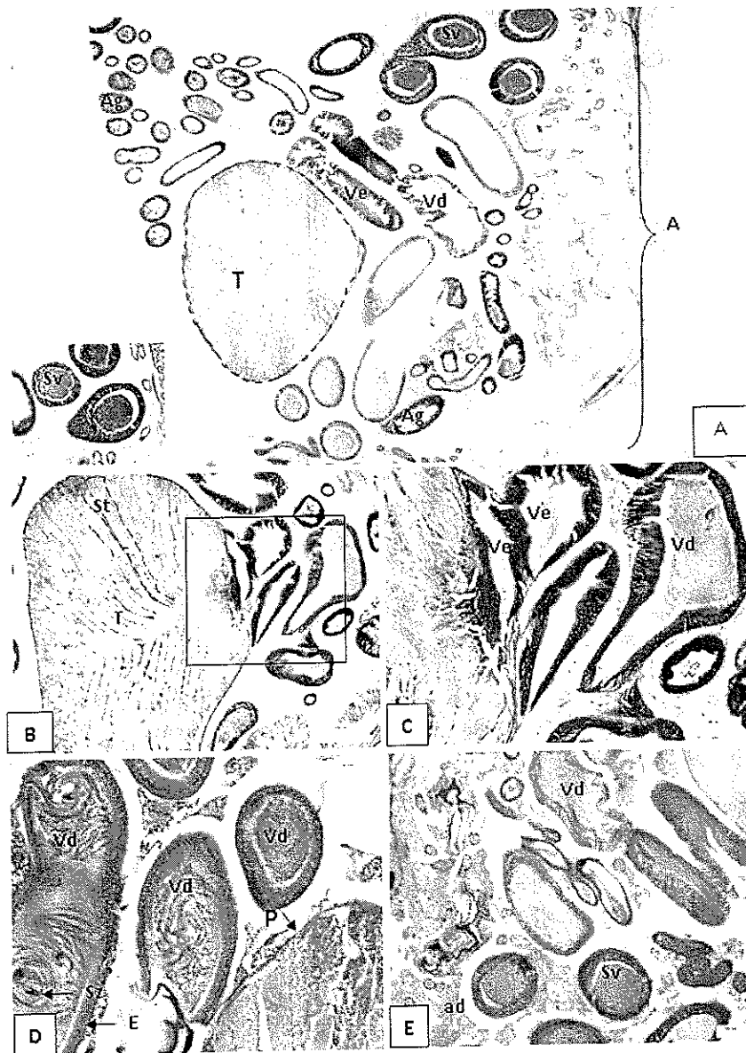
รูปที่ 1 ระบบสืบพันธุ์เพศผู้ : (A-E) ภาพตัดตามยาว แสดงรายละเอียดของระบบสืบพันธุ์เพศผู้ซึ่งประกอบด้วย อัณฑะ (T = testis) ท่อนำอสุจิ (Ve = vas efferens) ท่อนำอสุจিরวม (Vd = vas deferens) ต่อมเกี๋ยกูดเพศ (Ag = accessory gland) และต่อมสร้างน้ำเลี้ยงอสุจิ (seminal vesicle = Sv) (A-C = H&E, D-E = PAS) (A = abdomen, Sz = spermatozoa, E = epithelium, P = peritoneal membrane, ad = adipose tissue, Sv = seminal vesicle, St = Sperm tube)
