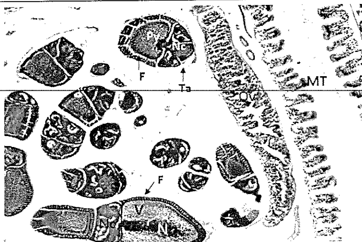
รูปที่ 3 ระบบสืบพันธุ์ของผีเสื้อหนอนคูนเพศเมีย : ภาพตัดตามยาวแสดงรายละเอียดของเซลล์ไข่ (ovary) ระยะต่าง ๆ ที่ถูกห่อหุ้มด้วยถุงห่อหุ้มโอวาริโอไล (tunica albuginea, Ta) และระยะต่าง ๆ ของเซลล์สืบพันธุ์ (H&E) (Pv = previtellogenic, V = vitellogenic, Y = yolk granule, MT = midgut, Ov = oviduct, Nc = nurse cell, F = follicular cell, N = nucleus)
