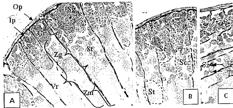
รูปที่ 2 ระยะโครงสร้างอวัยวะและระยะเซลล์สืบพันธุ์ : (A-C) ภาพตัดตามยาวของอัณฑะ (testis) ฝัเสื้อหนอนคูน เพศผู้ถูกหุ้มด้วยถุงห่อหุ้มอัณฑะชั้นนอก (outer peritoneal membrane, Op) และถุงห่อหุ้มอัณฑะชั้นใน (inner peritoneal membrane, Ip) ภายในอัณฑะประกอบด้วยหลอดสร้างอสุจิ (sperm tube) ซึ่งสังเกตเห็นระยะต่าง ๆ ของเซลล์สืบพันธุ์ (H&E) (Vr = vitellarium, Gr = germarium, Zg = zone of growth, Zm = zone of maturation, Zt = zone of transformation, Sg = spermatogonia, Sc = spermatocytes, St = spermatid, Sz = spermatozoa, H = head, T = tail)
